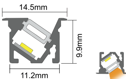
Dimensões
